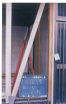
筋かいによる 補強
