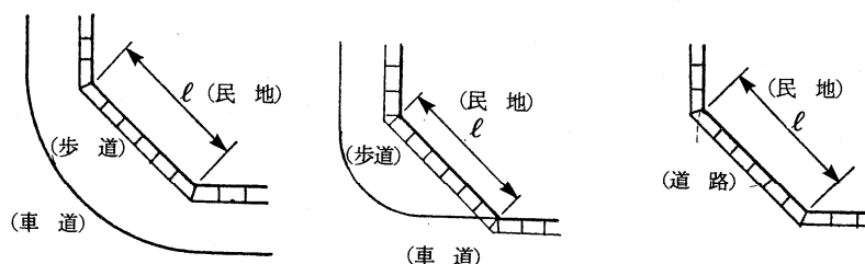
図 3.12 歩道の有無による隅切り方法
