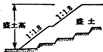
図 6 - 6 盛 土 高
