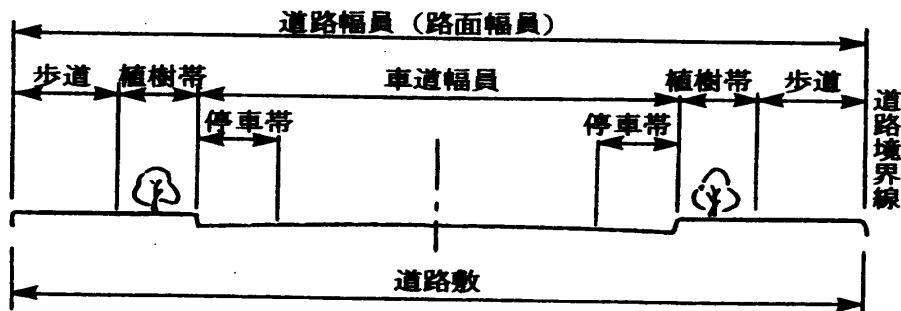
図 3.5 歩道等を設ける場合
