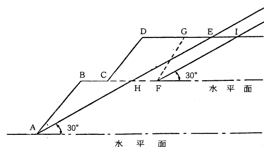
図 6.5 がけの範囲
