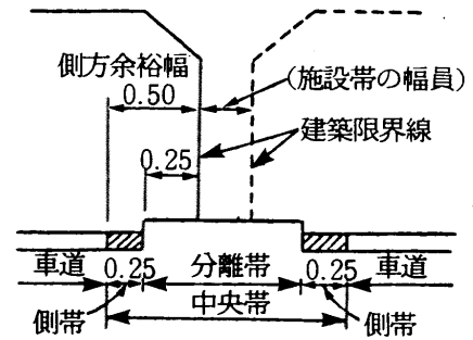
図3.10 中央帯の幅員構成
