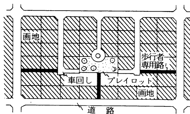
図2.3 袋路型
