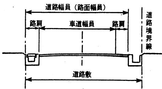
図 3.2 U型側溝の場合
