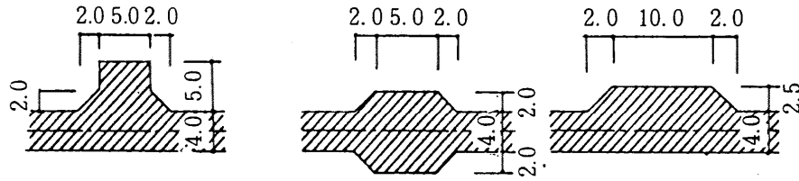
図 3.14 転回広場の規模（中間）
