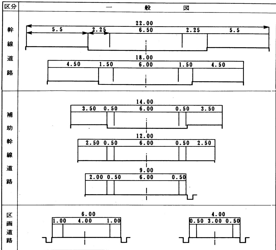
図 3.6 道路種別にみる分類
