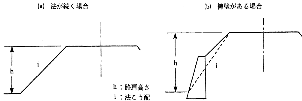
図 3.16 路肩高さ と 法勾配
