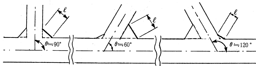
図 3.11 交差角度による隅切り方法
