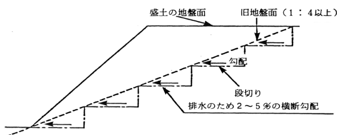
図 6.2 段 切 り
