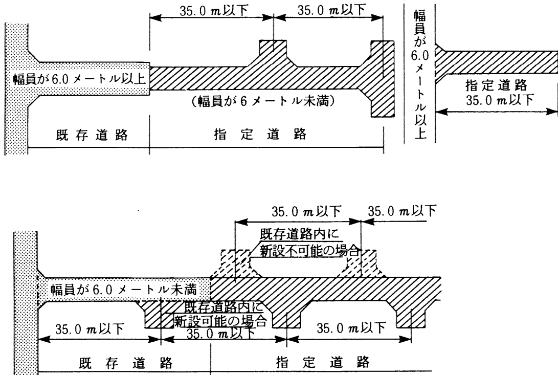
図 3.13 転回広場の間隔
