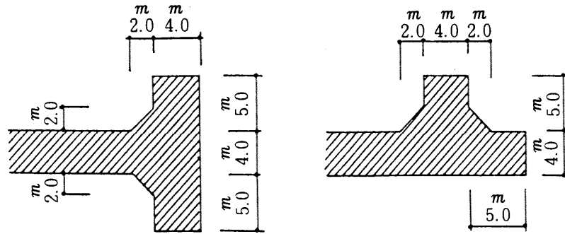
図 3.15 転回広場の規模（終端）
