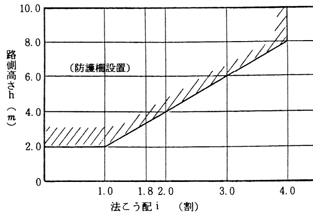
図 3.17 防護柵設置の範囲
