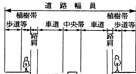
図3.9 植樹帯を設ける場合
