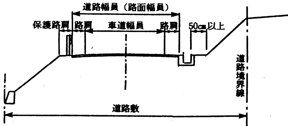
図 3.4 防護柵を設ける場合
