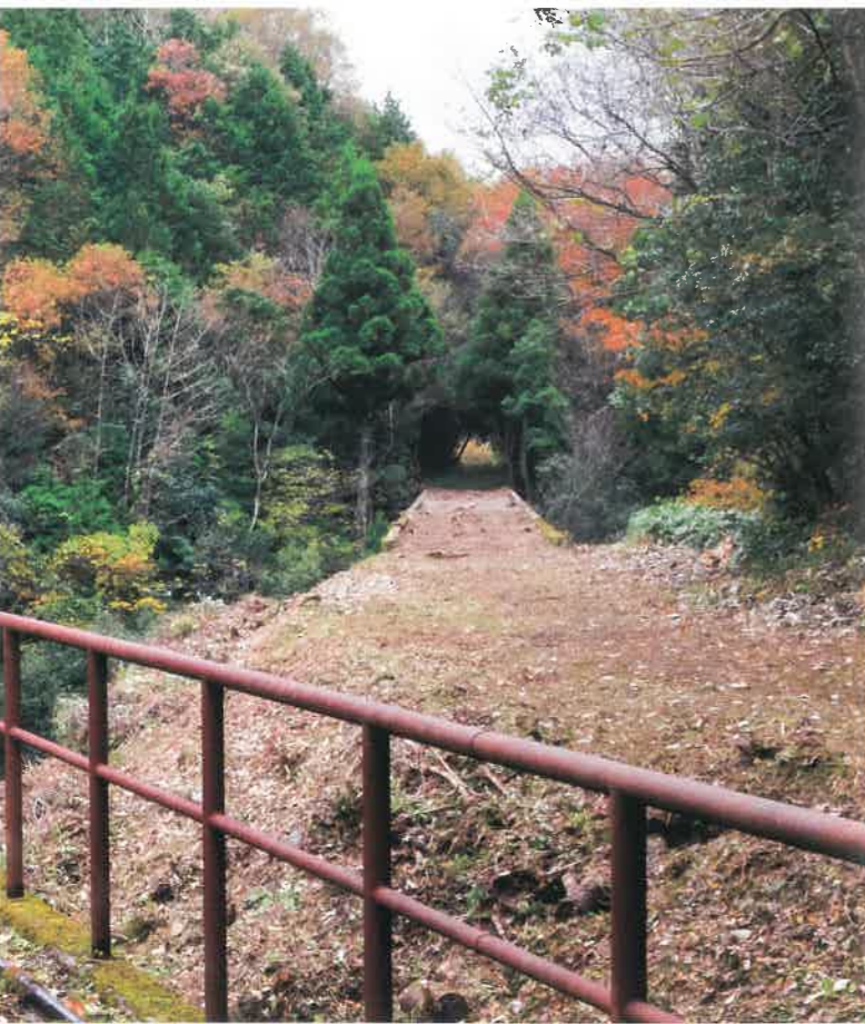
第一下府川橋梁と4連アーチ橋 新線旧線の橋梁が同時に見られる全国でも珍しいスポット。新線の第一下府川橋梁(写真左側)は、奥の下長屋トンネルへとつながっています。
