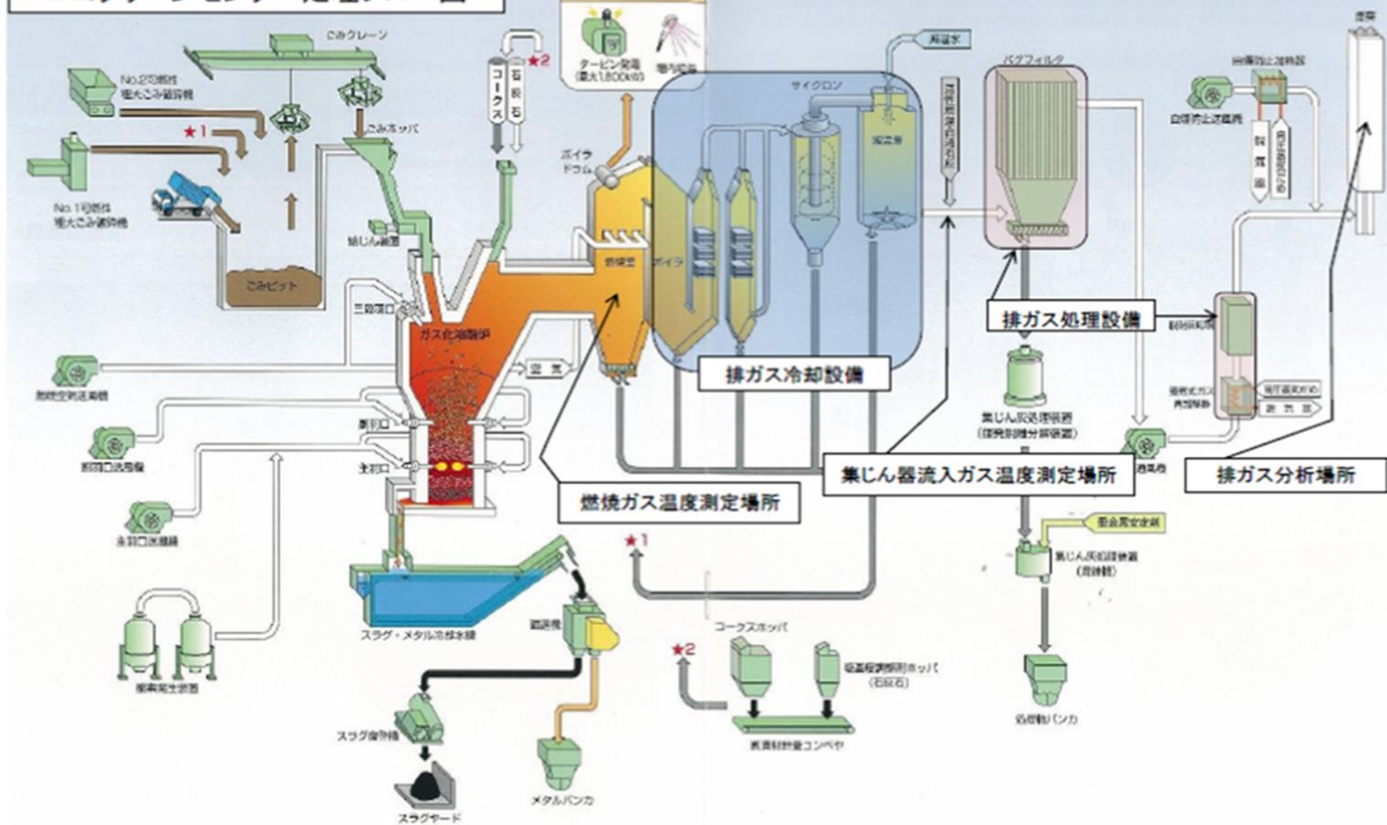
エコクリーンセンター処理フロー図
