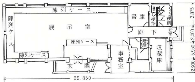
(一階平面図)
