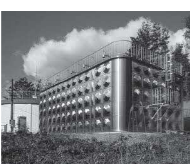
断水防止対策（今福地区増設タンク）
