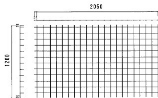
溶接金網 詳細図
