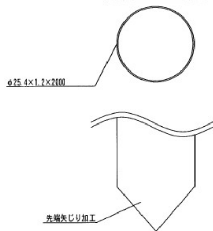
鋼管支柱 詳細図
