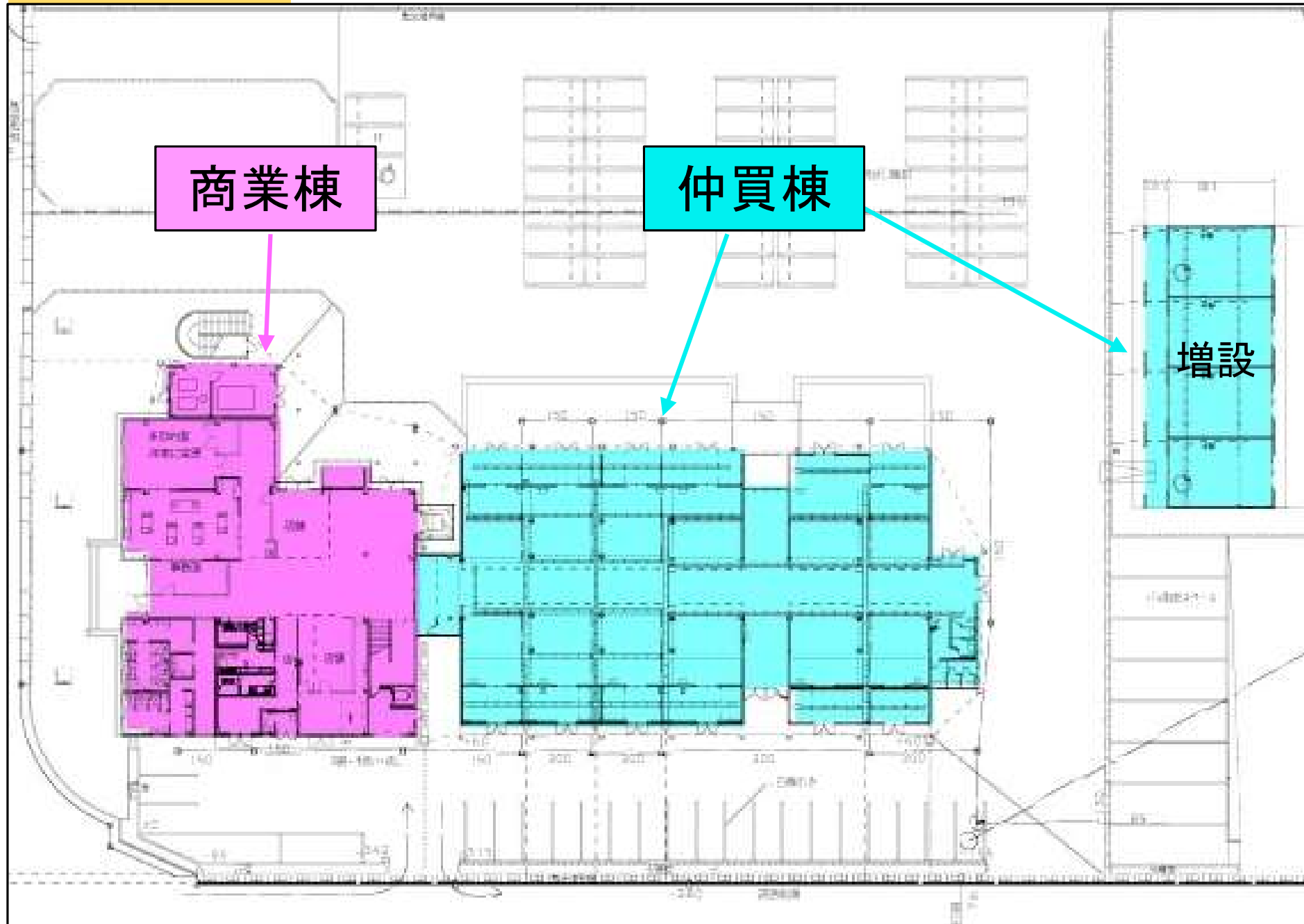
1階配置図
