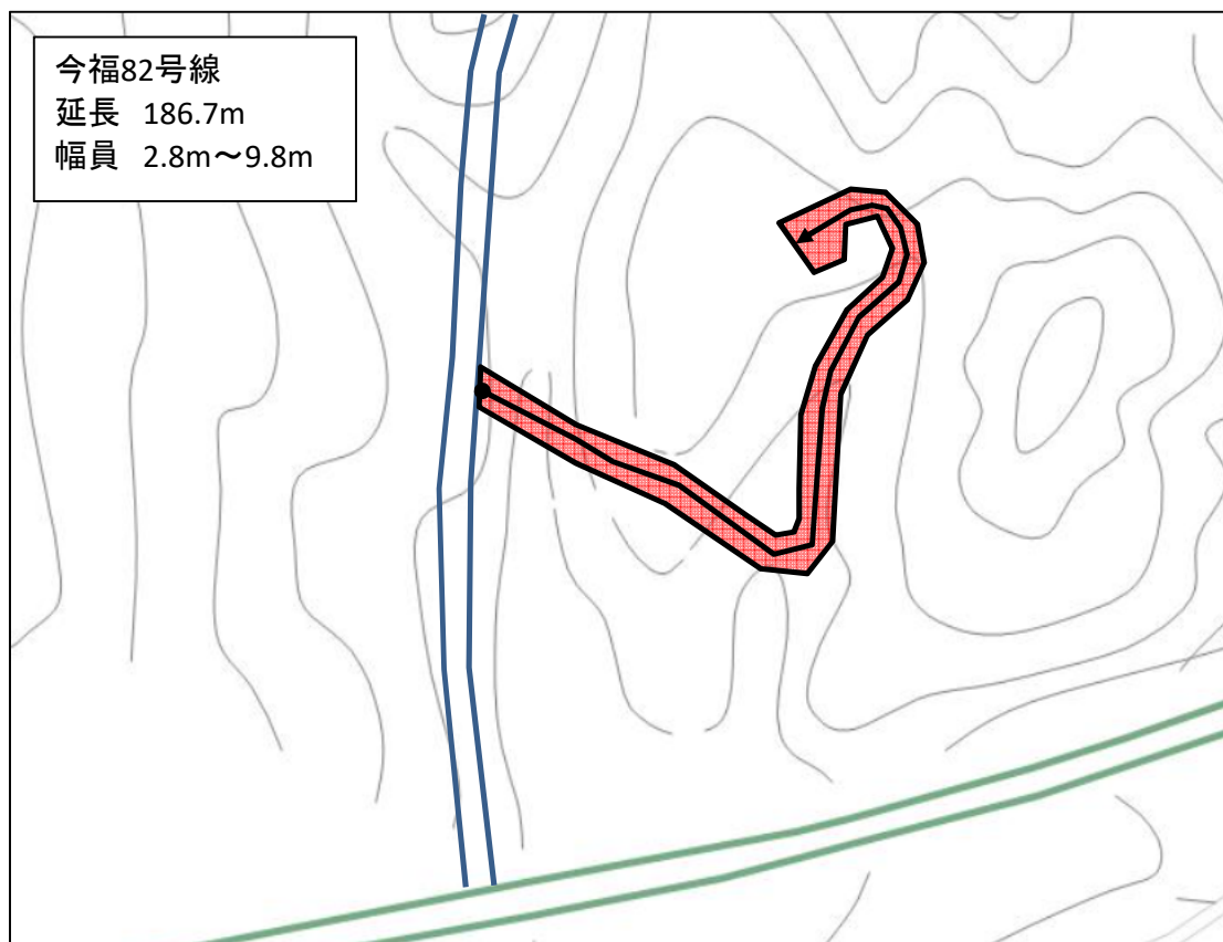
詳細図
